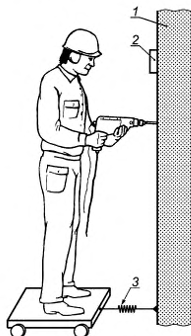
1 — бетонная стена; 2 — устройство считывания силы нажатия; 3 — динамометр
