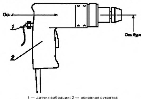
Рисунок 1 — Пример расположения датчика вибрации и направления измерений
