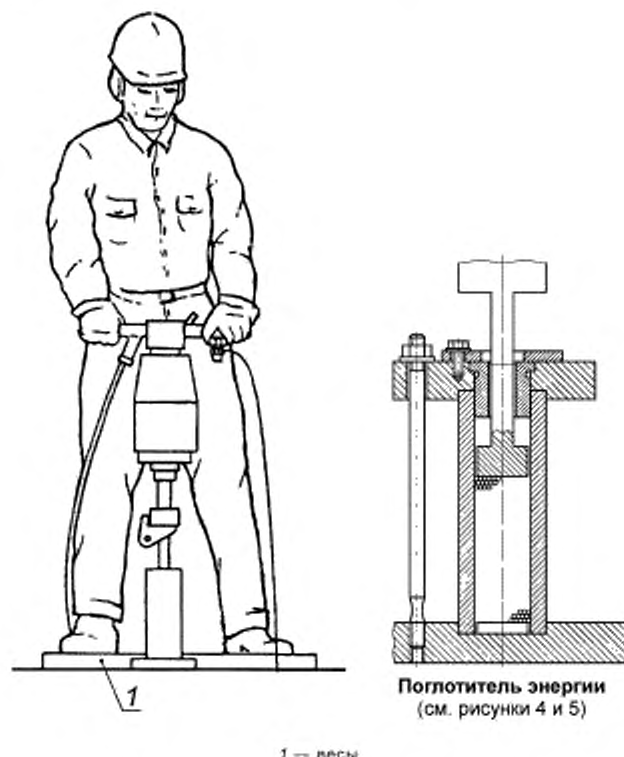
Рисунок 2 — Рабочая поза оператора при испытаниях бетонолома
