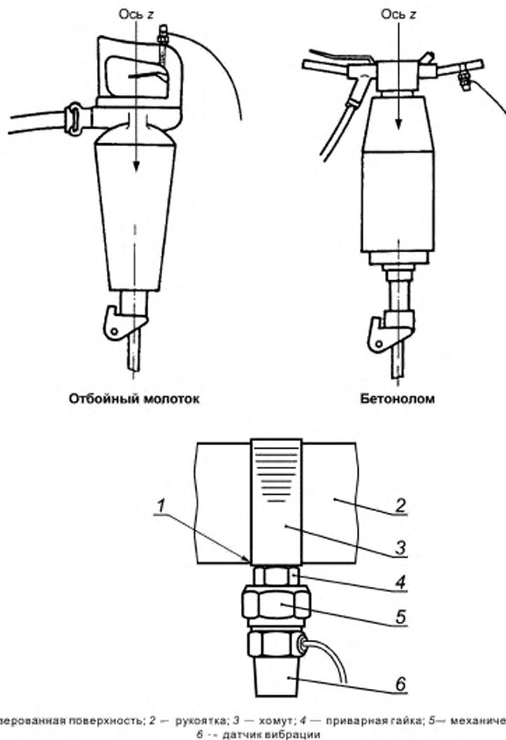
Рисунок 1 — Способы крепления датчика вибрации и направление измерений
