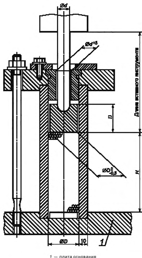
1 — плита основания
