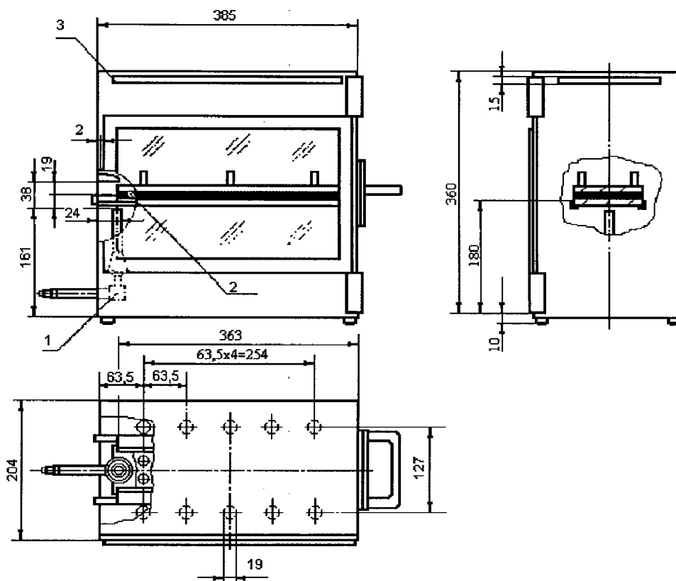
1 – газовая горелка; 2 – образец; 3 – вентиляционная прорезь
