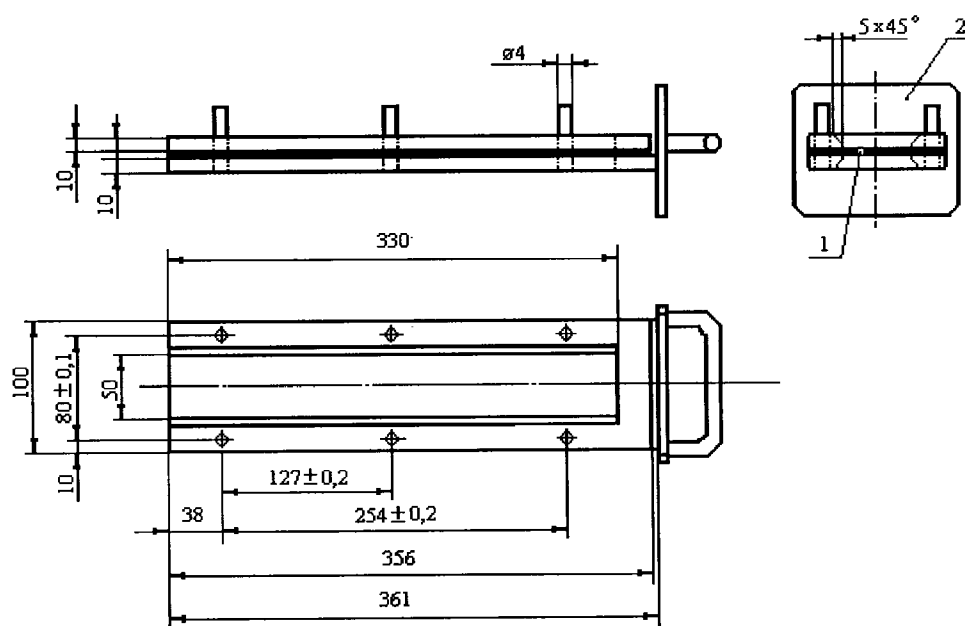
Рисунок 4 – Держатель образца с образцом
