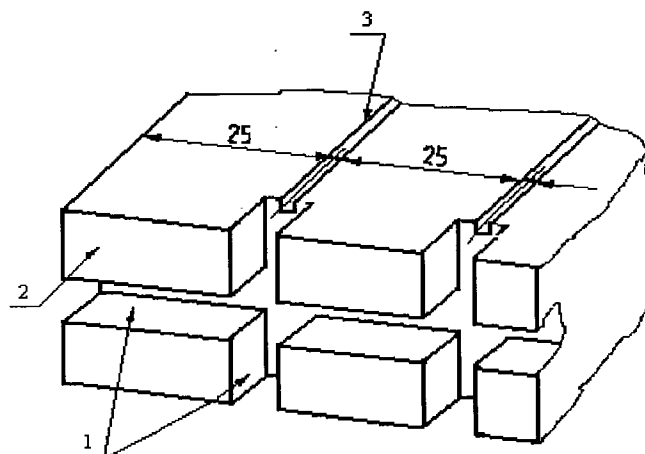
1 – выемка размером 2 \times 2 ; 2 – внешняя сторона рамки; 3 – выемка размером 0,5 \times 0,5
