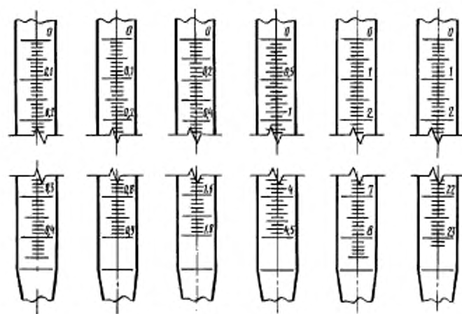
Градуировка и оцифровка пипеток с временем ожидания 15 с
