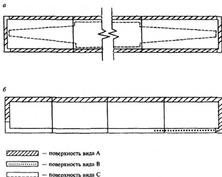
Рисунок 8 — Примеры определения видов поверхностей щитовых заготовок дверной фигурной филенки (а) и подоконной доски (б)
