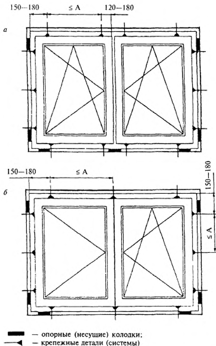
a — оконный блок с вертикальным импостом; б — оконный блок с безимпостным (штульповым) притвором; A — расстояние между крепежными деталями
