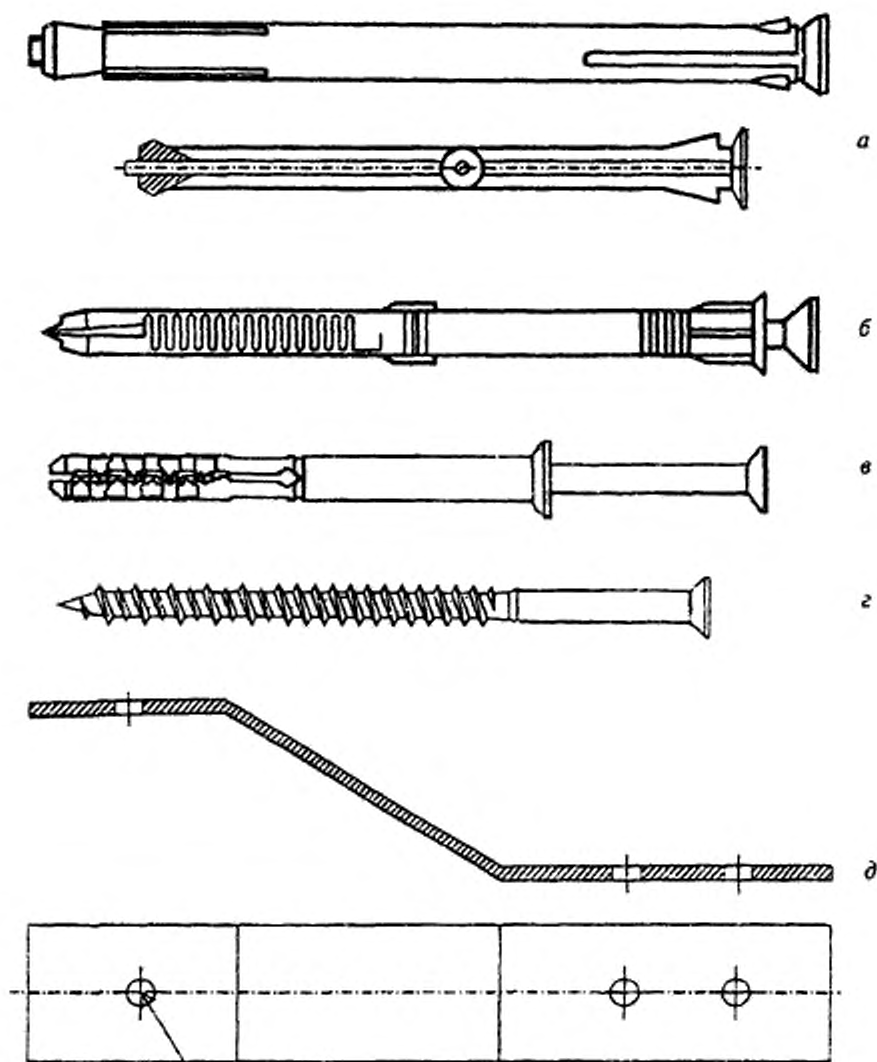
a — металлический рамный дюбель; b — пластмассовый рамный дюбель; v — универсальный пластмассовый дюбель со стопорным шурупом; z — строительные шурупы; d — гибкая анкерная пластина
