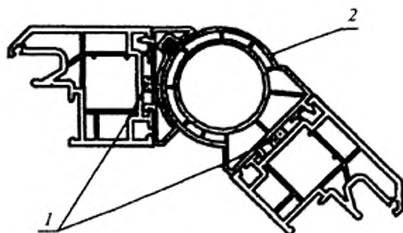
1 — изоляционная саморасширяющаяся паропроницаемая лента; 2 — угловой соединитель
