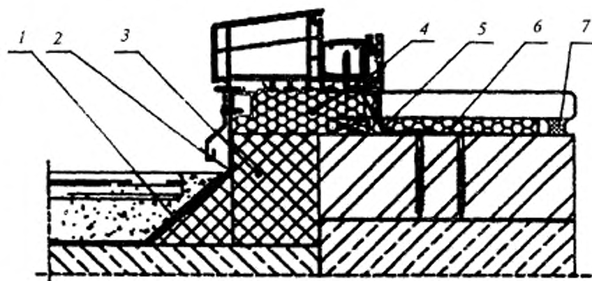
1 — водоизоляционная лента; 2 — водоизоляционная паропроницаемая лента; 3 — вкладыш из материала с низкой теплопроводностью; 4 — пенный утеплитель; 5 — пароизоляционная лента; 6 — гибкая анкерная пластина; 7 — герметик
