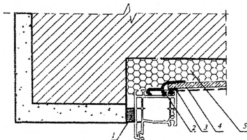
Рисунок А.12 — Монтажный шов в нижнем узле примыкания оконной коробки, подоконника и отлива в проеме однослойной стены
