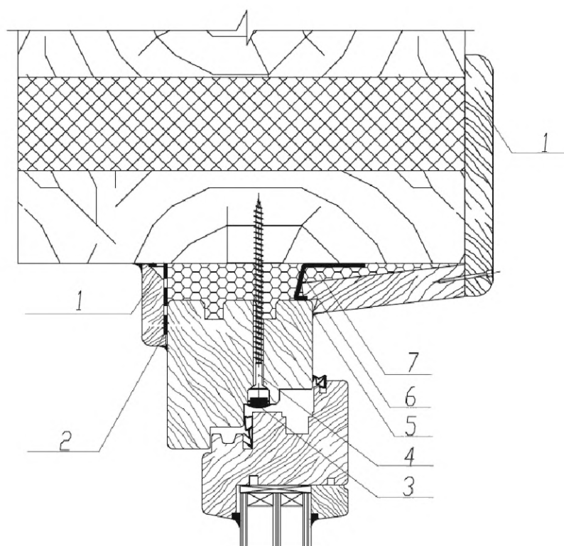
6 1 – нащельник; 2 – паропроницаемый герметик; 3 – декоративная заглушка; 4 – строительный шуруп; 5 – силиконовый герметик; 6 – пароизоляционный герметик; 7 – пенный утеплитель
