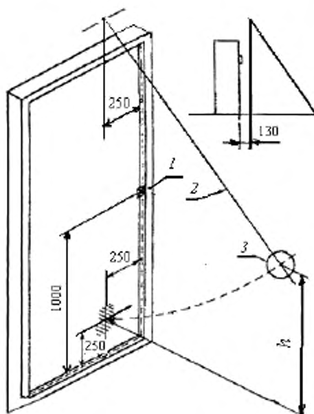
Рисунок Г.4 – Схема проведения испытания на сопротивлению удару мягким неупругим телом (грузом) в направлении открывания дверного полотна
