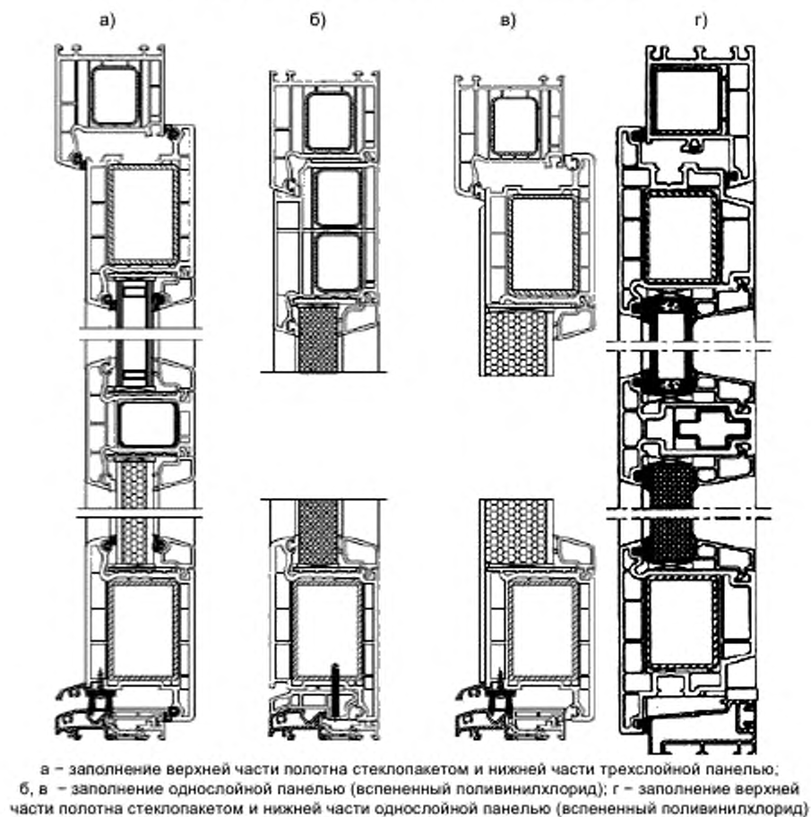
Рисунок Б.1 – Виды заполнения дверных полотен
