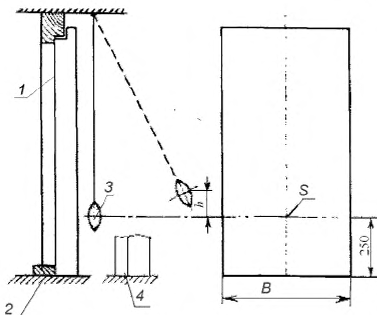
Рисунок Г.3 – Схема проведения испытания на сопротивлению удару мягким неупругим телом (грузом) в направлении закрывания дверного полотна
