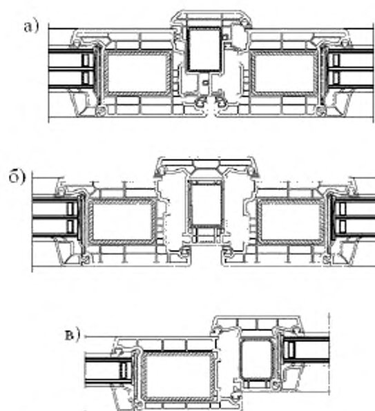
а) impostный притвор; б) штурьповой притвор; в) срединный притвор открывающихся и неоткрывающихся элементов Рисунок 3 – Примеры узлов срединных притворов дверных полотен
