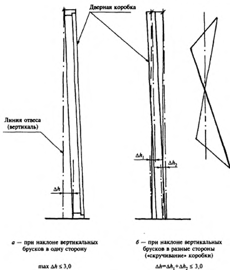
Рисунок В.2 — Определение отклонений дверной коробки
