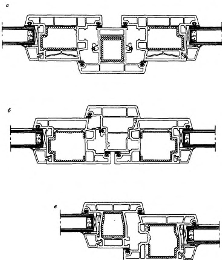
а — импостный притвор; б — штуповой притвор; в — срединный притвор открывающихся и неоткрывающихся элементов
