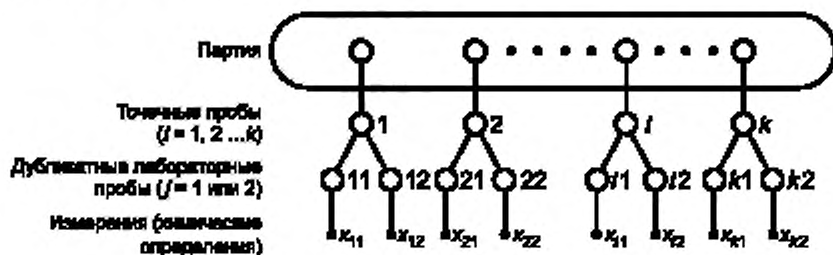
Рисунок 1 — Схема, применяемая к легкодробимым ферросплавам (вид I)
