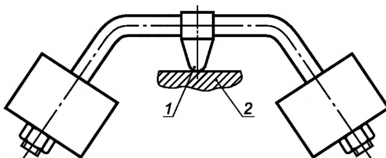
Рисунок 37 — Установка для испытания прочности материалов при нагревании
