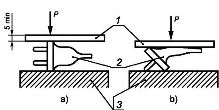
Рисунок 8 — Установка для испытания на сжатие
