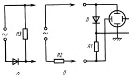
Схема измерения обратного тока (метод осциллографа)
