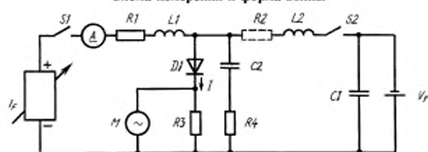
Схема измерения и форма волны
