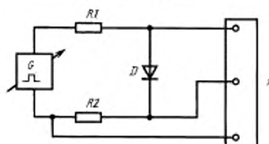
Схема измерения
