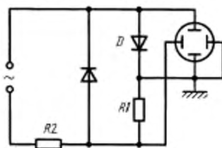
Схема измерения прямого напряжения (метод осциллографа)
