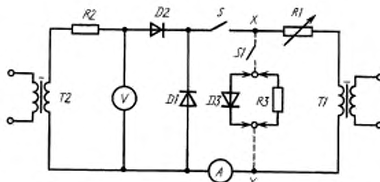
Схема измерения
