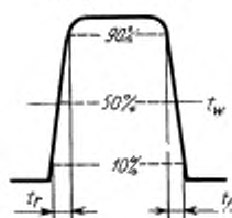
Форма волны
