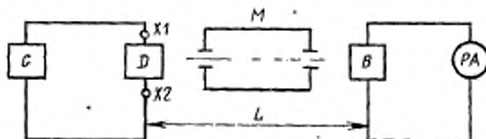
Г—генератор тока; D—излучатель (проверяемый или образцовый); X1, X2—контакты подключения излучателя; M—спектральный прибор; В—фотоприемник; РА—измеритель тока; L—расстояние от излучателя до фотоприемника
