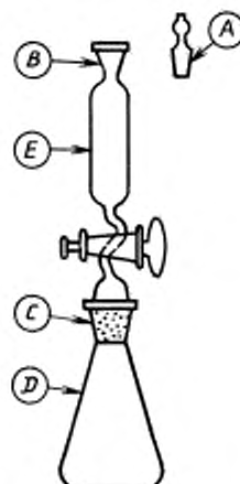
Аппарат для определения потребления хлора целлюлозой
