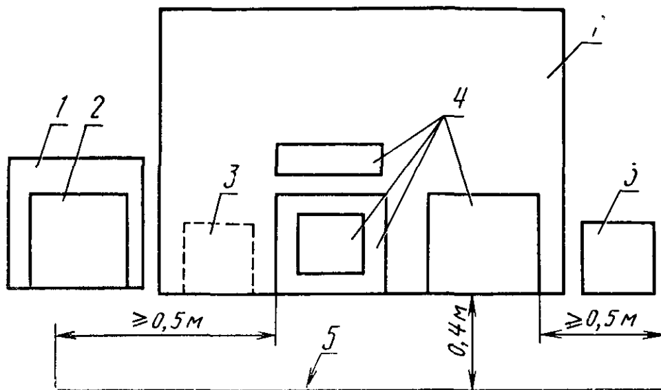
Пример расположения аппаратуры и оборудования при измерении напряжения радиопомех, создаваемых настольными ТС (вид сверху)
