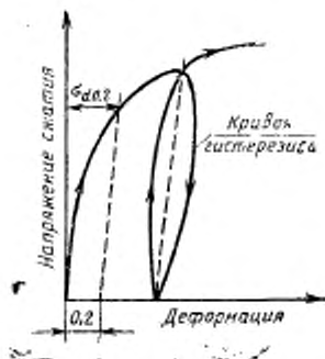
Черт. 2. Определение 0,2%-ного предела текучести при сжатии \sigma_{сж.2} с помощью линии, параллельной центральной линии кривой гистерезиса, на расстоянии, соответствующем 0,2% деформации
