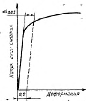
Черт. 1. Определение 0,2%-ного предела текучести при сжатии с помощью параллельной прямой Гука, проведенной на расстоянии, соответствующем 0,2% деформации
