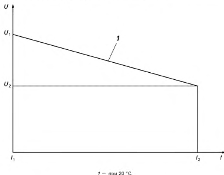
Рисунок 1 — Вольтамперная характеристика источника питания стартера
