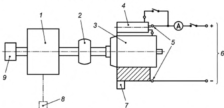
1 — тормоз переменной нагрузки; 2 — муфта; 3 — стартер; 4 — соленоид (втягивающее реле); 5 — выводы стартера; 6 — питание стартера; 7, 8 — точки измерения крутящего момента; 9 — измерение частоты вращения
