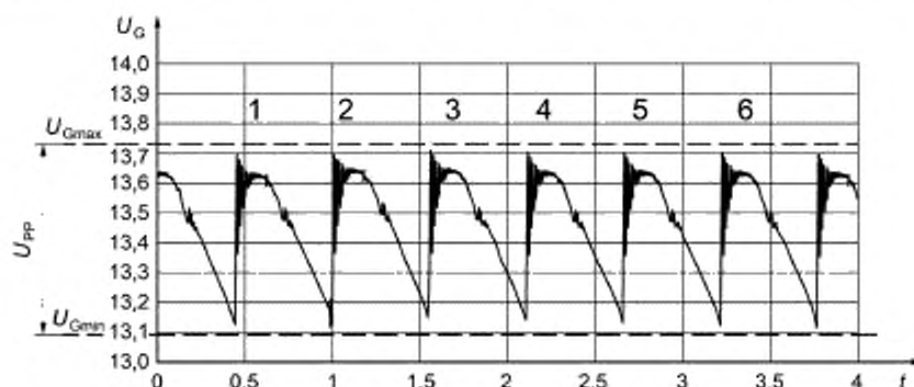
Рисунок 5 — Схематический вид колебаний напряжения ( p = 6 )
