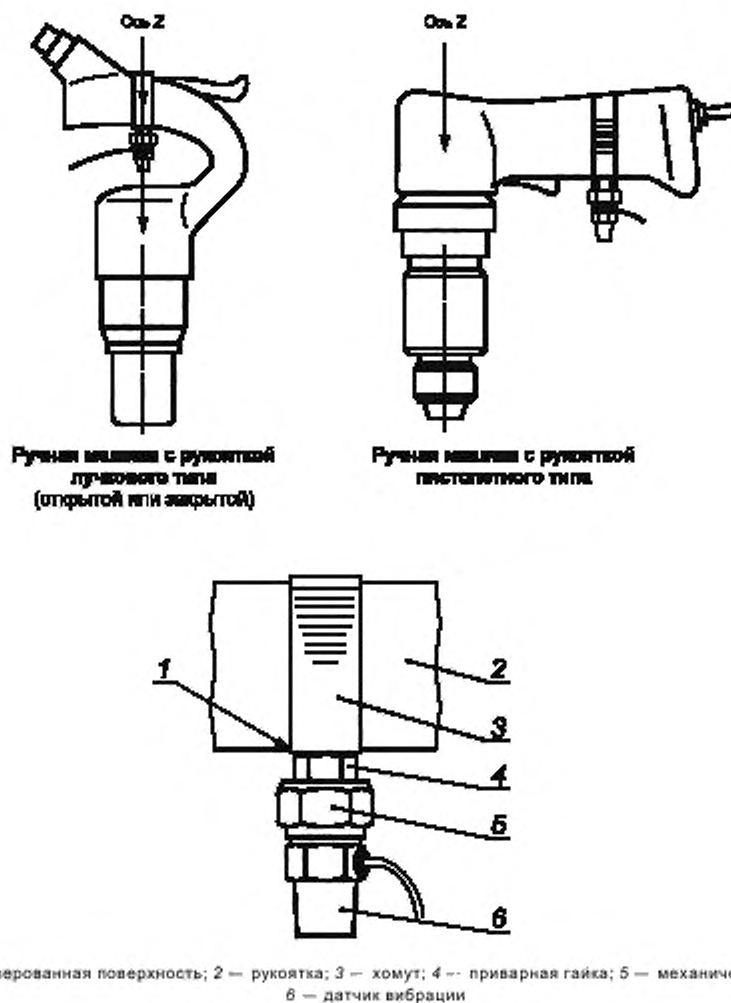
Рисунок 1 — Способы крепления датчика вибрации и направление измерений
