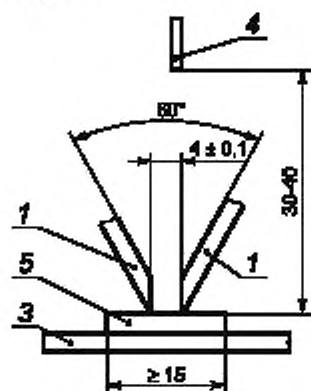
3 — опора; 4 — конец капиллярной; 5 — образец
