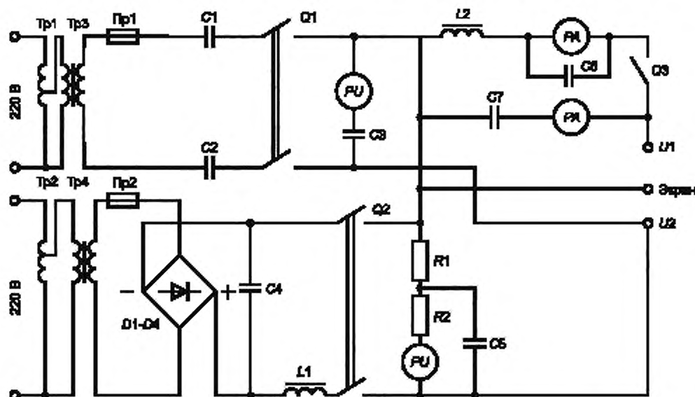
D1—D4 — диоды; Тр1, Тр2 — автотрансформаторы; Тр3, Тр4 — разделительные трансформаторы; Пр1, Пр2 — предохранители; Q1, Q2 — тумблеры; С1—С5 и С7 — бумажные конденсаторы (фильтры); С6 — конденсатор электролитический (фильтр); L1, L2 — дроссели (фильтры); R1, R2 — внутреннее сопротивление вольтметра; U1, U2 — измерительные выводы
