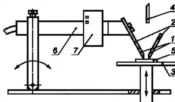
1 — платиновый электрод; 2 — медный удлинитель; 3 — опора; 4 — конец капиллярной; 5 — образец; 6 — изоляционная трубка; 7 — груз
