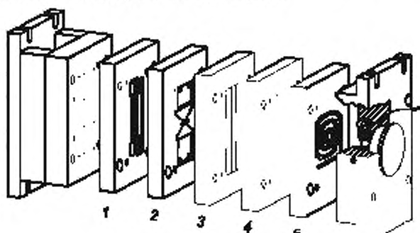
1, 2, 3, 4, 5 - сменные пластины формы для литья
