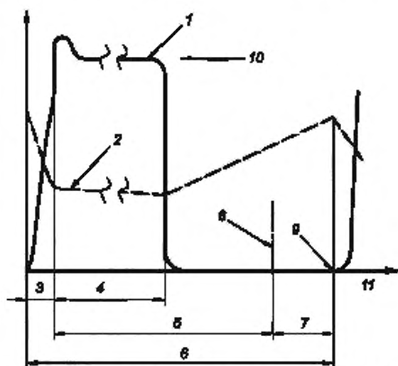
1 – давление на материал p ; 2 – продольное положение шнека. 3 – время лития t_i ; 4 – время остановки t_H , 5 – время отверждения t_{CR} ; 6 – время цикла t_T ; 7 – время открытия t_O ; 8 – открытие формы; 9 – закрытие формы, 10 – давление остановки p_H ; 11 – время
