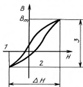
Импульсное возбуждение с постоянным подмагничивающим полем
