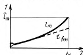
Нелинейность намагничивающего тока
