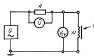
Схема цепи, в которой применяется измерительная катушка индуктивности
