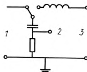
1 — регулируемый источник питания; 2 — контроль тока; 3 — испытательная обмотка
