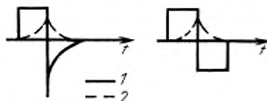
а) экспоненциальное восстановление
