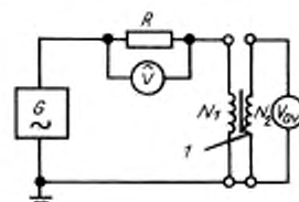
Схема цепи, в которой применяется измерительная катушка взаимной индуктивности
