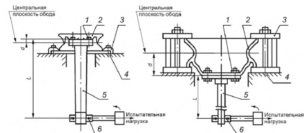
Колесо с профилем посадочной полки обода 5°
