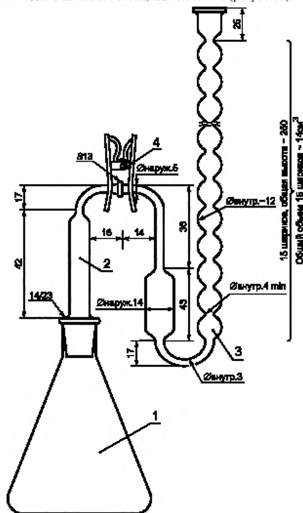
Рисунок 1 — Стеклянный прибор для отгонки и поглощения мышьяка
