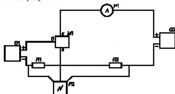
G1 — источник импульсного тока; G2 — источник постоянного напряжения; R1 , R2 — безиндуктивные измерительные резисторы с малым сопротивлением; P1 — измеритель амплитудных значений тока; P2 — осциллограф; M1 — испытуемый модуль
