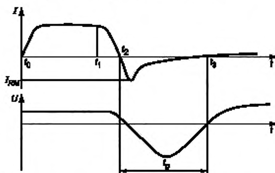
I_{RM} — импульсный обратный ток; t_g — время выключения
