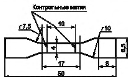
Рисунок 4 — Образец в форме двусторонней лопатки небольшого размера
