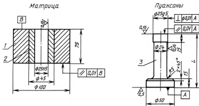
Схема пресс-формы для изготовления прессовок цилиндрической формы
