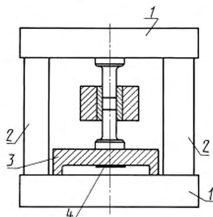
Схема пресс-формы
