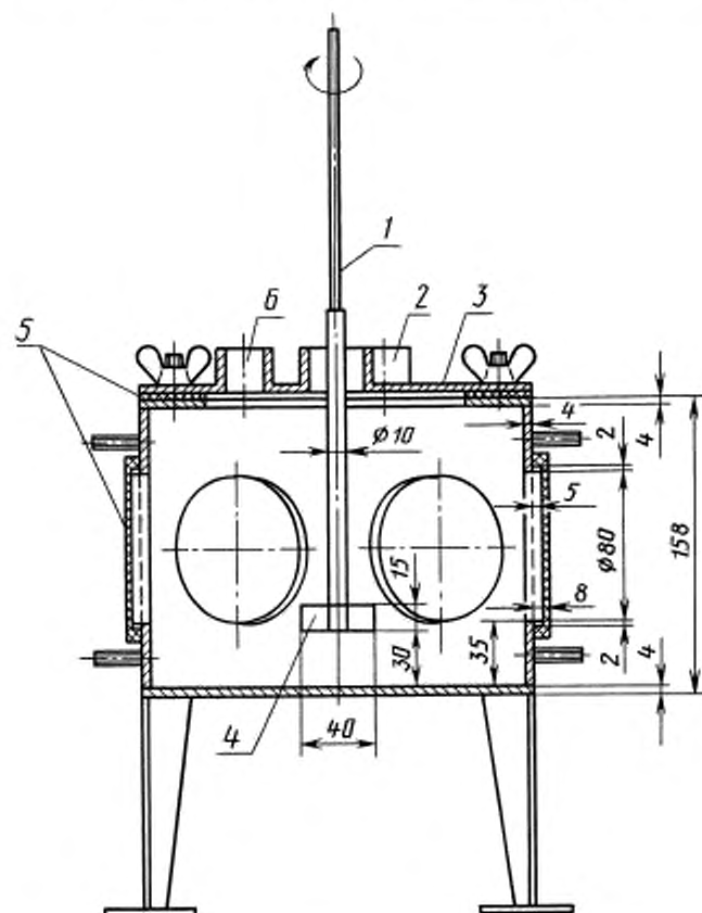
1 — мешалка с лопастями; 2 — отверстие для нагревателя погружения; 3 — крышка; 4 — толщина (2 мм); 5 — кольцо уплотнения; 6 — отверстие для устройства для регулирования температуры
