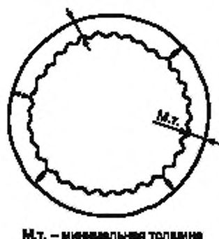
Рисунок 7 — Измерение толщины оболочки (внутренний круглый профиль неправильной формы)
