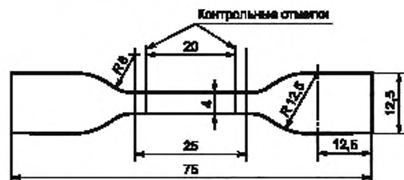
Рисунок 12 — Образец в виде двусторонней лопатки
