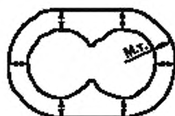
Рисунок 10 — Измерение толщины оболочки (двужильный плоский шнур в оболочке)
