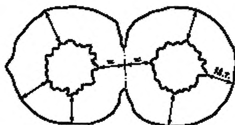
Рисунок 6 — Измерение толщины изоляции (двужильный плоский шнур без оболочки)
