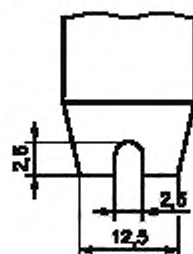
Рисунок 14 — Конец вырубного ножа с выемкой
