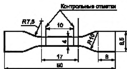
Рисунок 13 — Образец в виде лопатки уменьшенного размера
