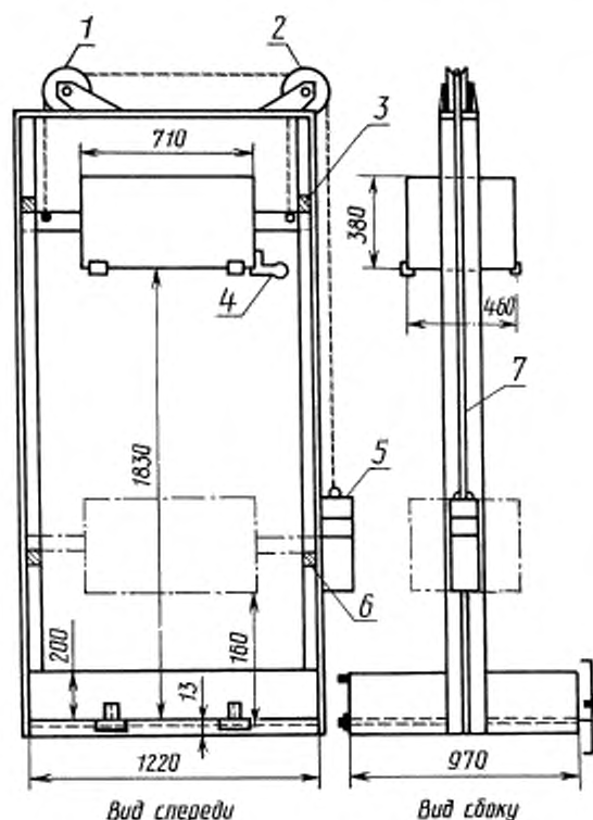
1 — одинарный шкив; 2 — двойной шкив; 3, 6 — столпы; 4 — защелка; 5 — противовес; 7 — направляющий паз
