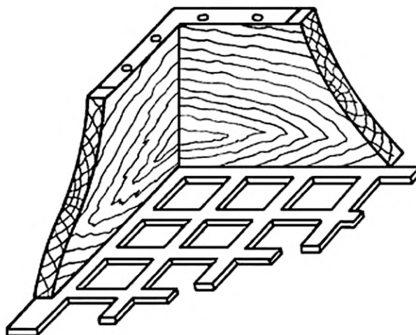
Рисунок 2 — Деталь сита
