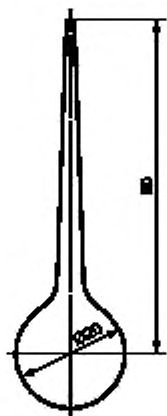
Рисунок 1 — Ампула стеклянная сферическая
