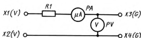
X1(V) , X2(V) — выводы для подключения прибора; R1 — ограничительный резистор; PA — микроамперметр; PV — вольтметр; X3(G) , X4(G) — выводы для подключения источника питания
