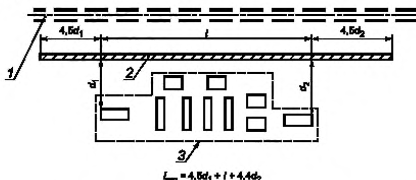
Рисунок 2 — Схема определения требуемой длины акустического экрана
