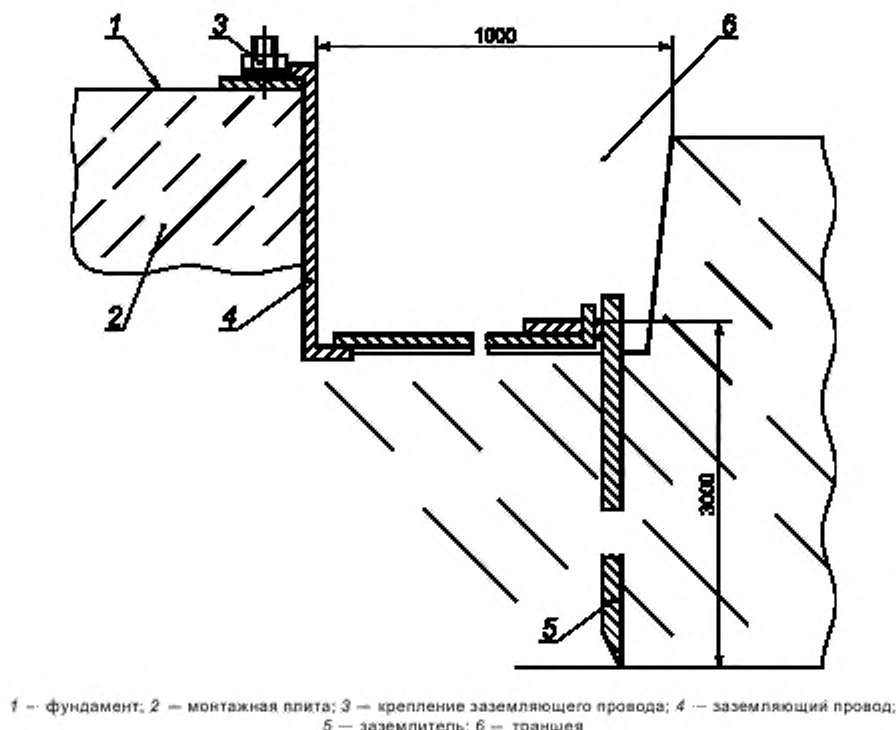
Рисунок 7 — Схема производства заземления
