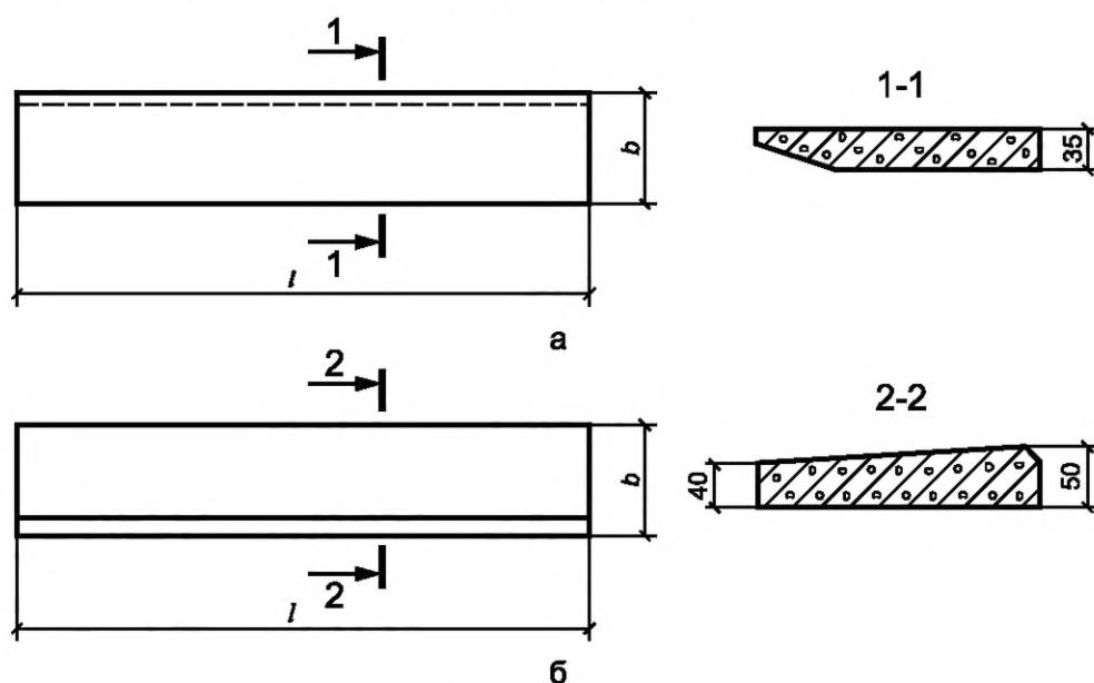
Рисунок 8 — Накладная проступь типа 1ЛН
