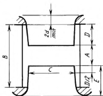
Тип 2. Конструкция барабана с ограждением ребра корпусом лебедки
