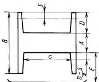
Тип 1. Конструкция пустого барабана
