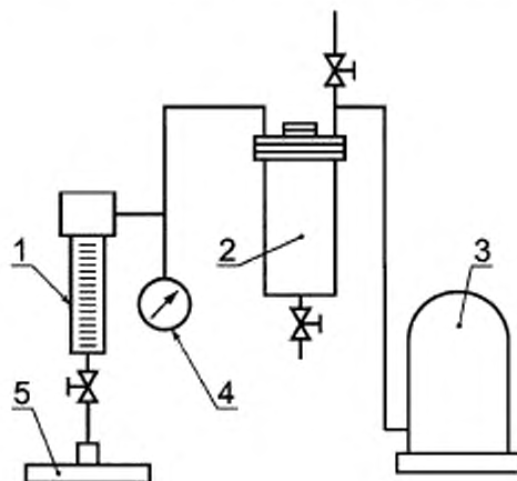
1 — фильтрационная колонка, выполненная из органического стекла, с фильтрационной перегородкой поверхностью 1 см 2 . Фильтрационная перегородка выполнена из нержавеющей штампованного сита с размером ячейки 100 мкм; 2 — напорный сосуд, выполненный из органического стекла; 3 — компрессор, предназначенный для создания необходимого постоянного давления в фильтрационной колонке; 4 — образцовый манометр для измерения давления в системе; 5 — подвижный столик с мерными цилиндрами
