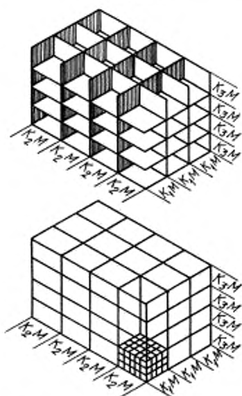
Прямоугольная модульная пространственная координационная система
