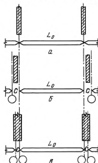
Расположение координационных осей в плане зданий с несущими стенами
