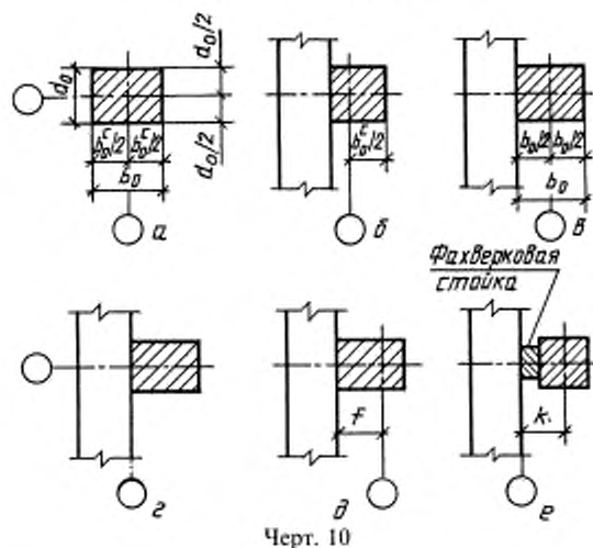
Привязка колонн каркасных зданий к координационным осям
