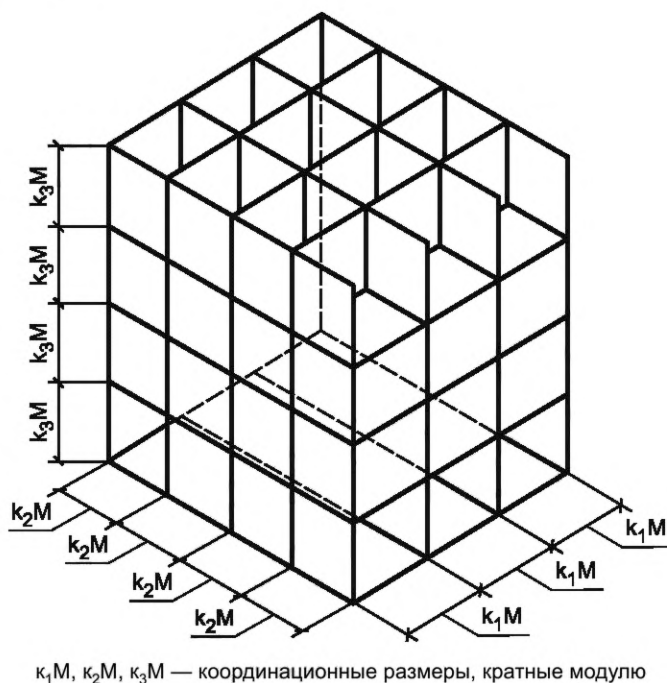
Рисунок 1 — Прямоугольная модульная координационная система
