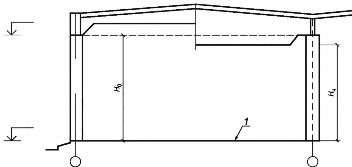
Рисунок 14 — Модульная (координатная) высота этажа одноэтажных зданий
