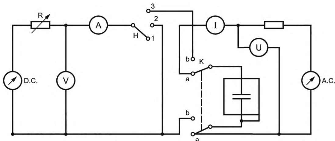
Рисунок 1 — Цепь для выполнения испытания на разрушение
