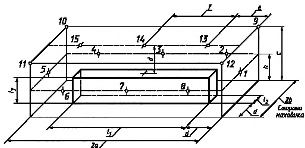
Рисунок 3 — Размещение пятнадцати точек измерений на измерительной поверхности
