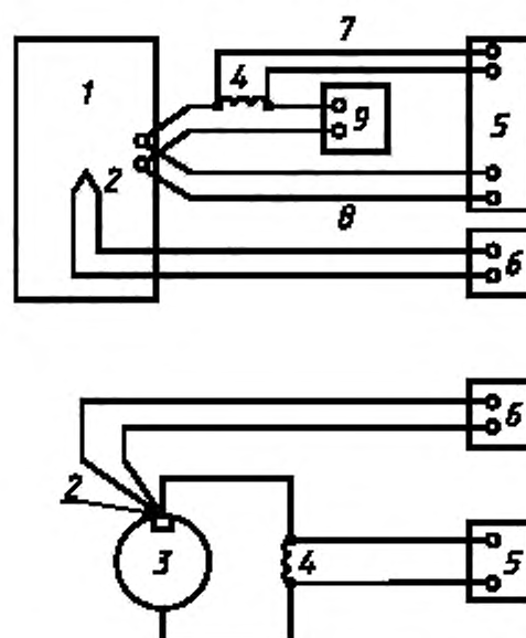
Измерительная схема
