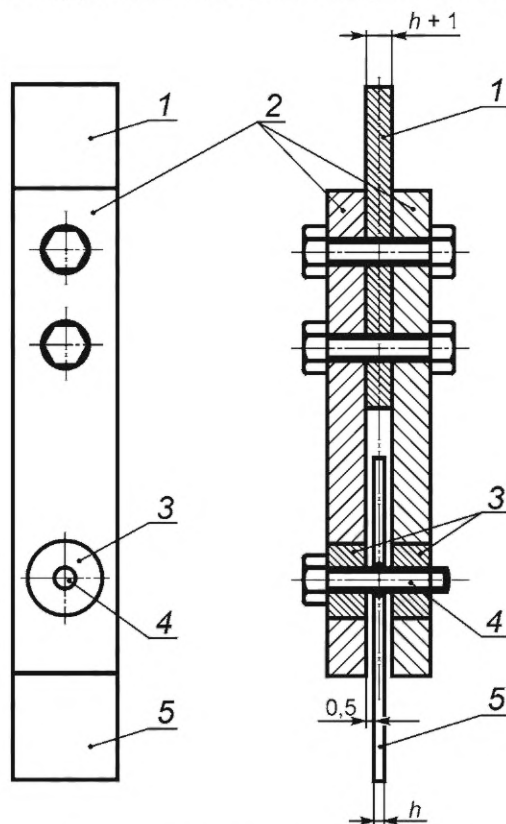
1 — распорная плита (толщина = h + 1 мм); 2 — боковая плита из закаленной стали; 3 — втулки из закаленной стали, посадка скольжения в боковых плитах (опционально); 4 — гладкий штифт; 5 — образец для испытаний
