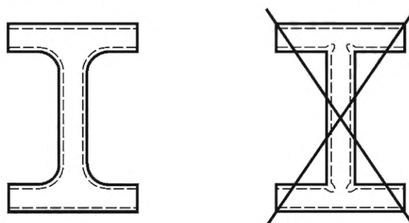
Рисунок Г.3 — Расположение мата в сечении
