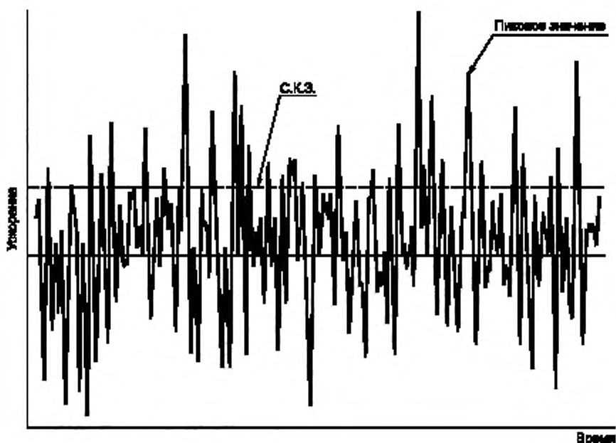
Рисунок A.2 — Отсечка (ограничение) сигнала
