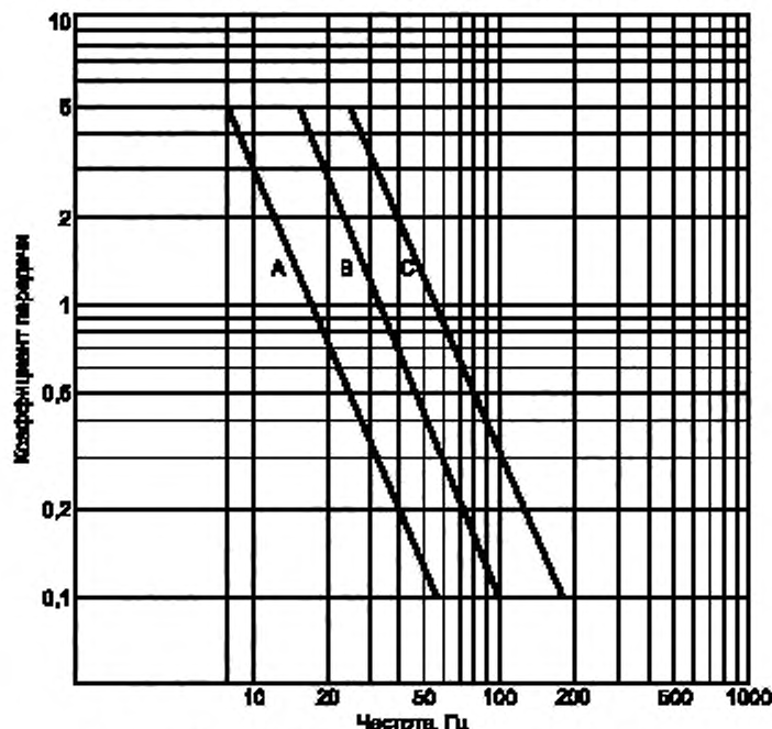
Рисунок А.6 — Коэффициент передачи виброизолятора
