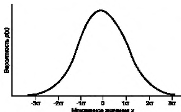
Рисунок A.1 — Гауссовская плотность распределения вероятностей
