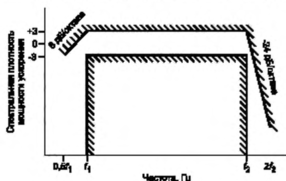
Рисунок 2 — Границы допуска для спектральной плотности мощности ускорения
