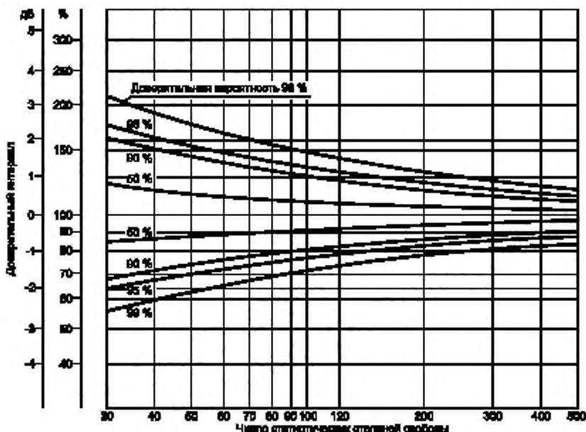
Рисунок A.4 — Доверительные интервалы оценки спектральной плотности мощности ускорения для различных значений доверительной вероятности в зависимости от числа статистических степеней свободы
