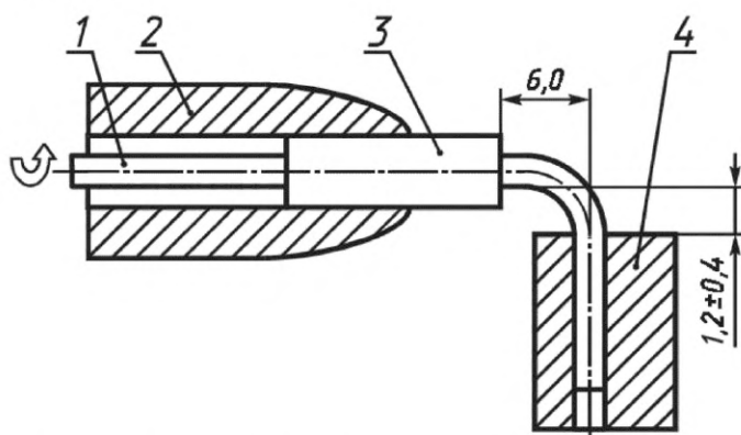
Рисунок 2 — Испытание с закрепленным корпусом изделия
