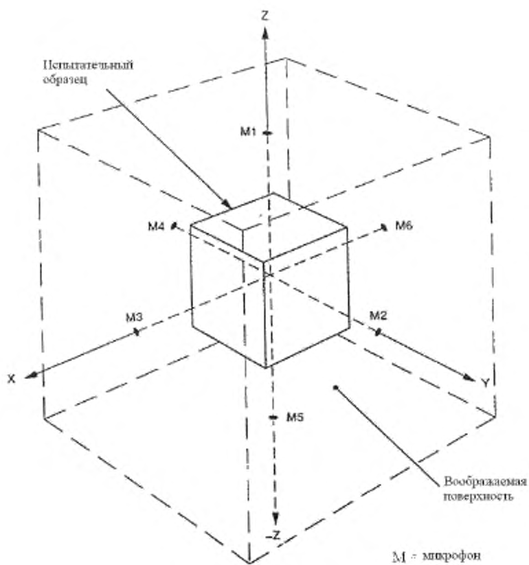
Рисунок 5 - Типовое расположение микрофонов контрольных точек (1-6) на восбрасываемой поверхности вокруг образца
