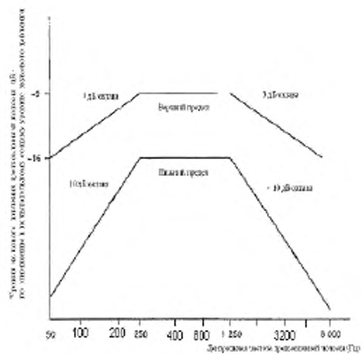
Рисунок 1. Спектр предельной частоты для вибрирующей системы
