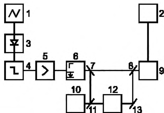
1 — осциллограф; 2 — испытуемое изделие; 3 — частотный детектор; 4 — ограничитель; 5 — полосуовой усилитель на частоту 30 МГц; полоса пропускания 0,5 МГц; 6 — фотоэлектронный умножитель; 7, 8, 11 — полупрозрачные зеркала (с коэффициентом отражения не менее 50 %); 9 — фокусирующая система; 10 — газовый оптический квантовый генератор; 12 — устройство для сдвига частоты; 13 — зеркало с коэффициентом отражения не менее 90 %
