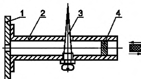
1 — диафрагма; 2 — волновод (10 × 23); 3 — антенна; 4 — поршень настройки
