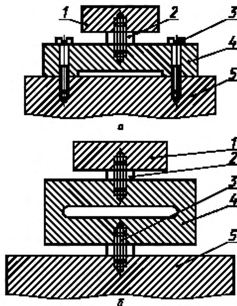
a — крепление балки к столу стенда в двух точках; б — крепление балки к столу стенда в одной точке
