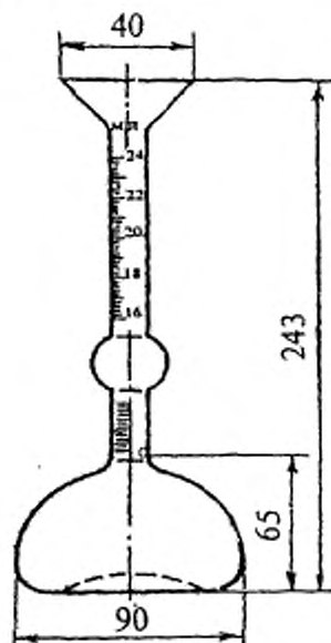
Рисунок 1 — Прибор Ле-Шателье
