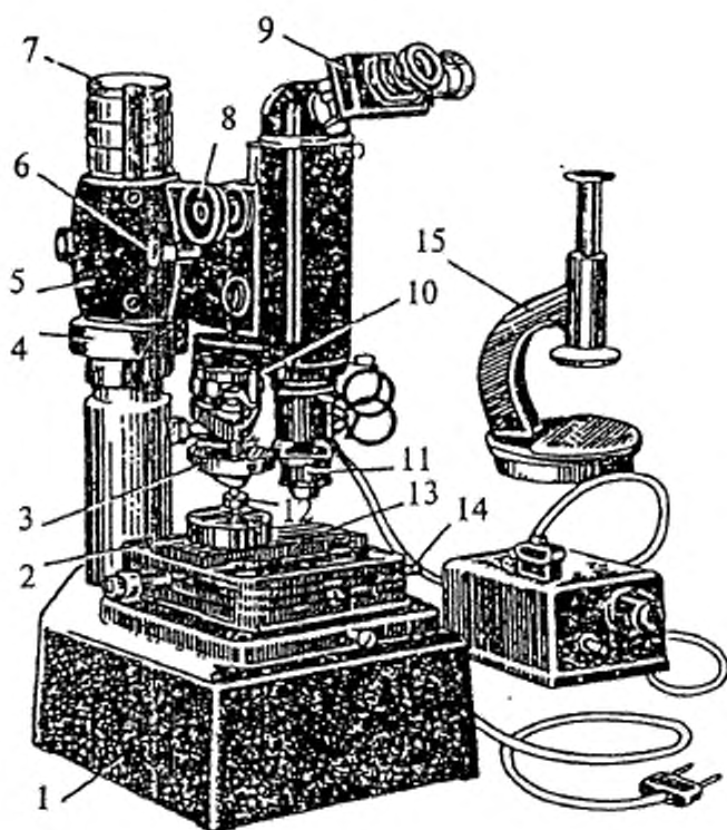
1 — основание прибора; 2 — предметный столик; 3 — гиря из разновеса; 4 — гайка для перемещения кронштейна с брусом; 5 — кронштейн бруса; 6 — барашек микрометрического движения; 7 — колонка; 8 — барашек грубого движения; 9 — винтовой окулярный микрометр; 10 — рукоятка арретира; 11 — объектив; 12 — оправка с алмазным наконечником; 13 — планка для закрепления исследуемого образца; 14 — рукоятка для поворота столика; 15 — ручной прессик
